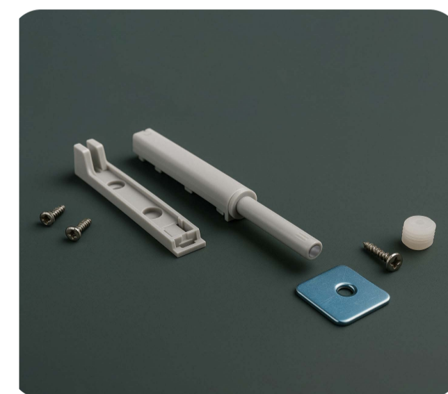
KT push gris con imán + placa adhesiva con tornillo + base.
